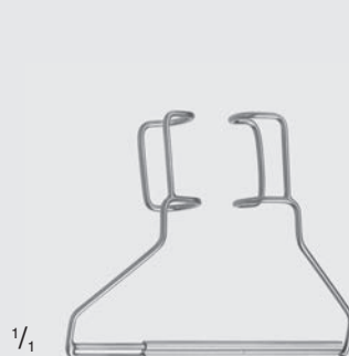
H-1067B Barraquer-Oosterhuis Lidsperrer, gefenstert, verstellbar, für Kinder Eye speculum, fenestrated, adjustable, baby size Blefaróstato, fenestrado, ajustable, para niños Blépharostat, fenêtré, ajustable, pour enfants
